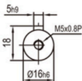
Arbre type S2 shaft
