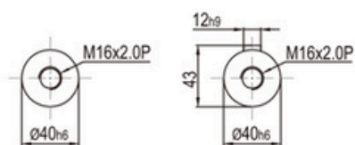
Arbre type S2 shaft
