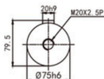
Arbre type S2 shaft
