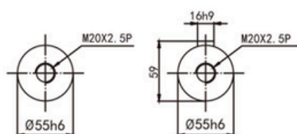
Arbre type S1 shaft
