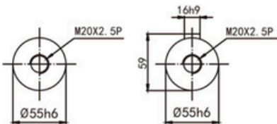
Arbre type S2 shaft
