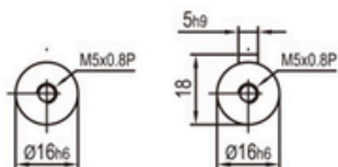
Arbre type S1 shaft
